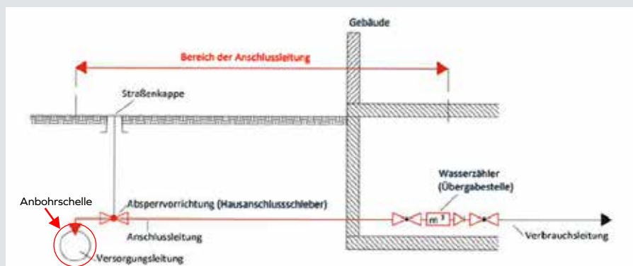
Die Eigentümer sind für den roten Bereich verantwortlich (Anbohrschelle, Absperrventil, Anschlussleitung).
